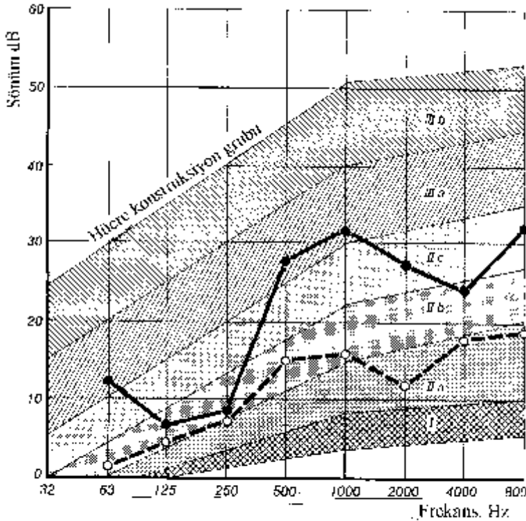
Şekil 7 : Çeşitli tip hücrelerin ses sönümü ve açıklıkların bu etkisi
