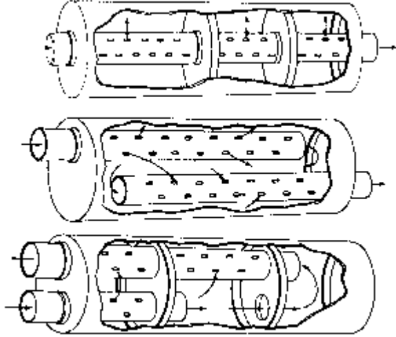
Şekil 9. Reaktif susturucu örnekleri
