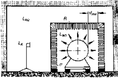
Şekil 6 - Ses kaynağı makinelerin hücre içine alınması
