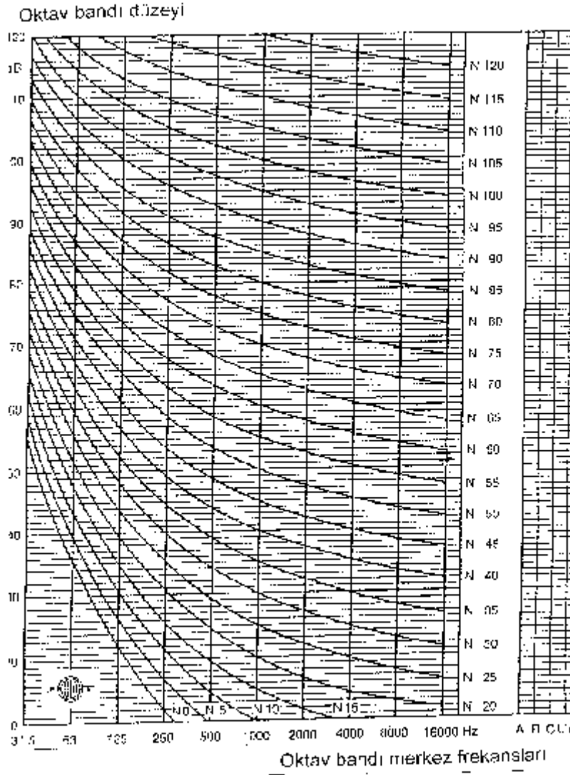
Şekil 3. NC eğrileri
