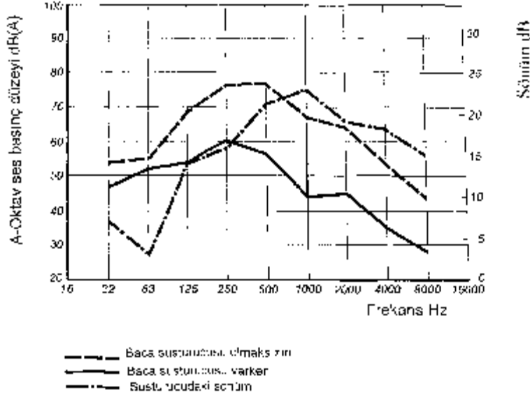
Şekil 15. Örnek baca susturucusu sönüm deneyi sonuçları
