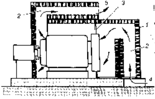
Şekil 8 : Bir elektrik motoru Labirent hava giriş çıkış açıklıkları.
